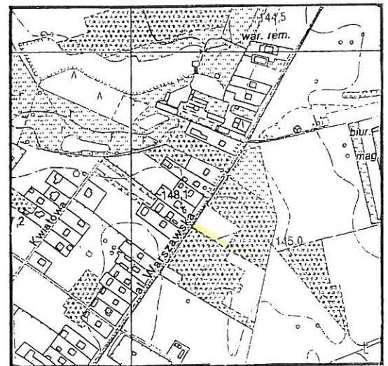
Szkie lokalizacyjny w skali 1: 10 000
