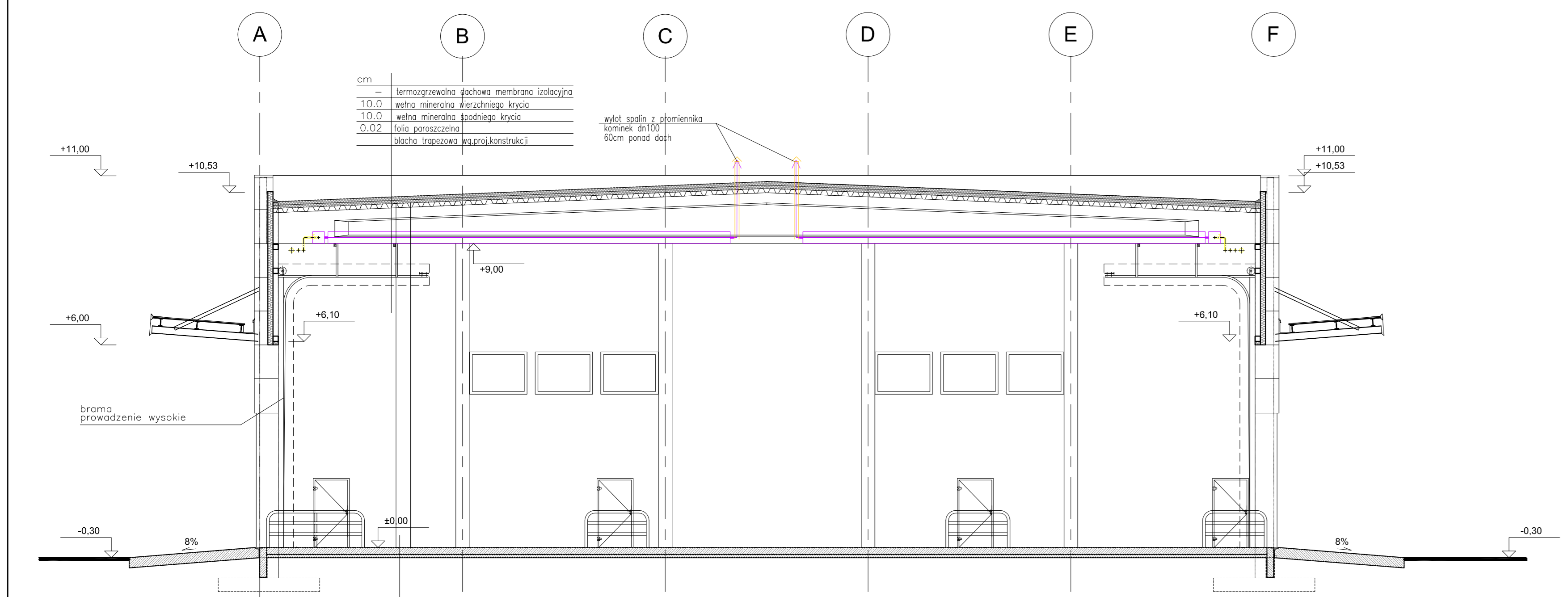
PRZEKRÓJ 8-8 SKALA 1:100
