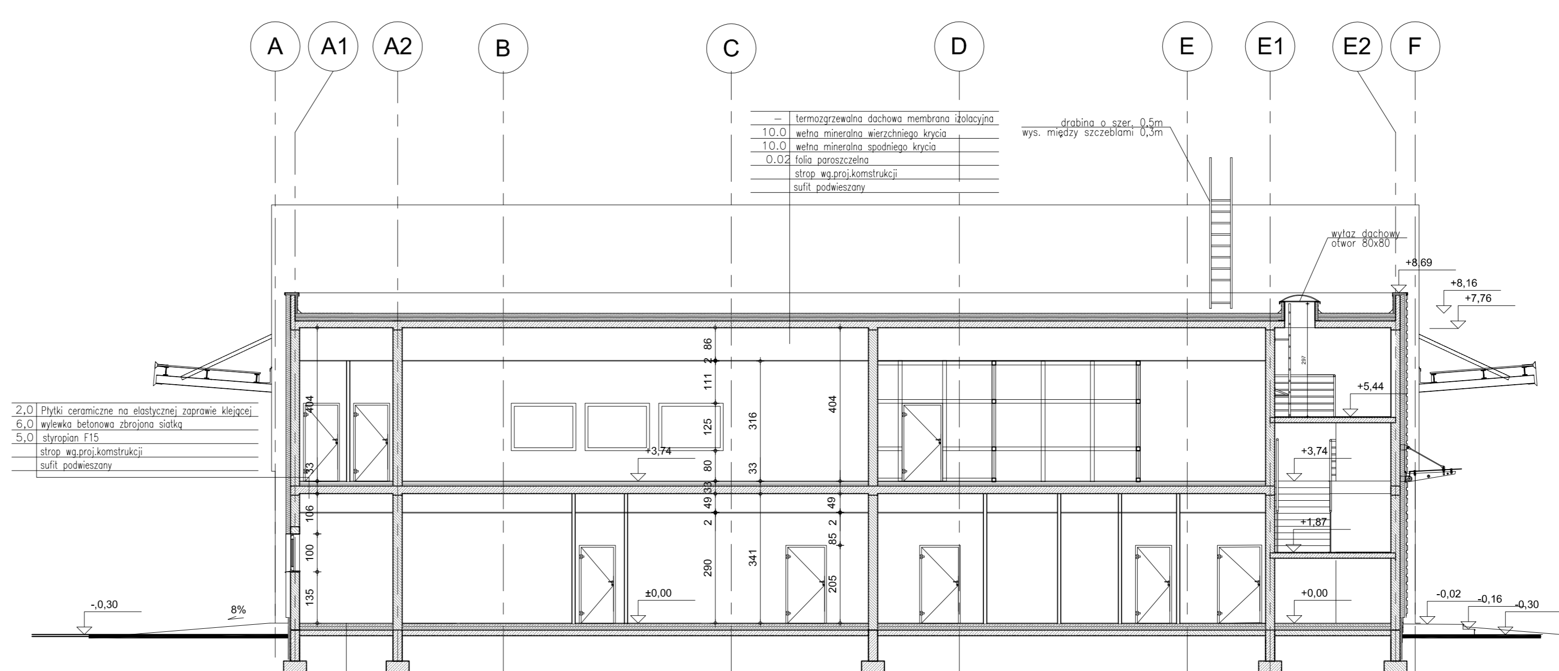
PRZEKRÓJ 1-1 SKALA 1:100
