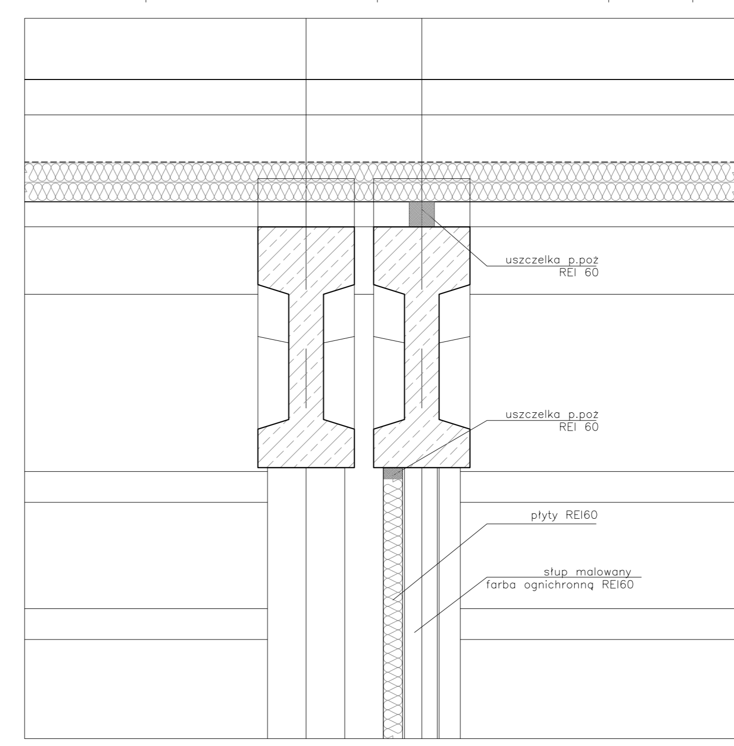
DETAL A SKALA 1:20
